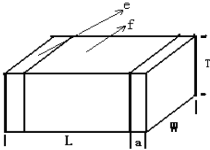
外形尺寸图:
